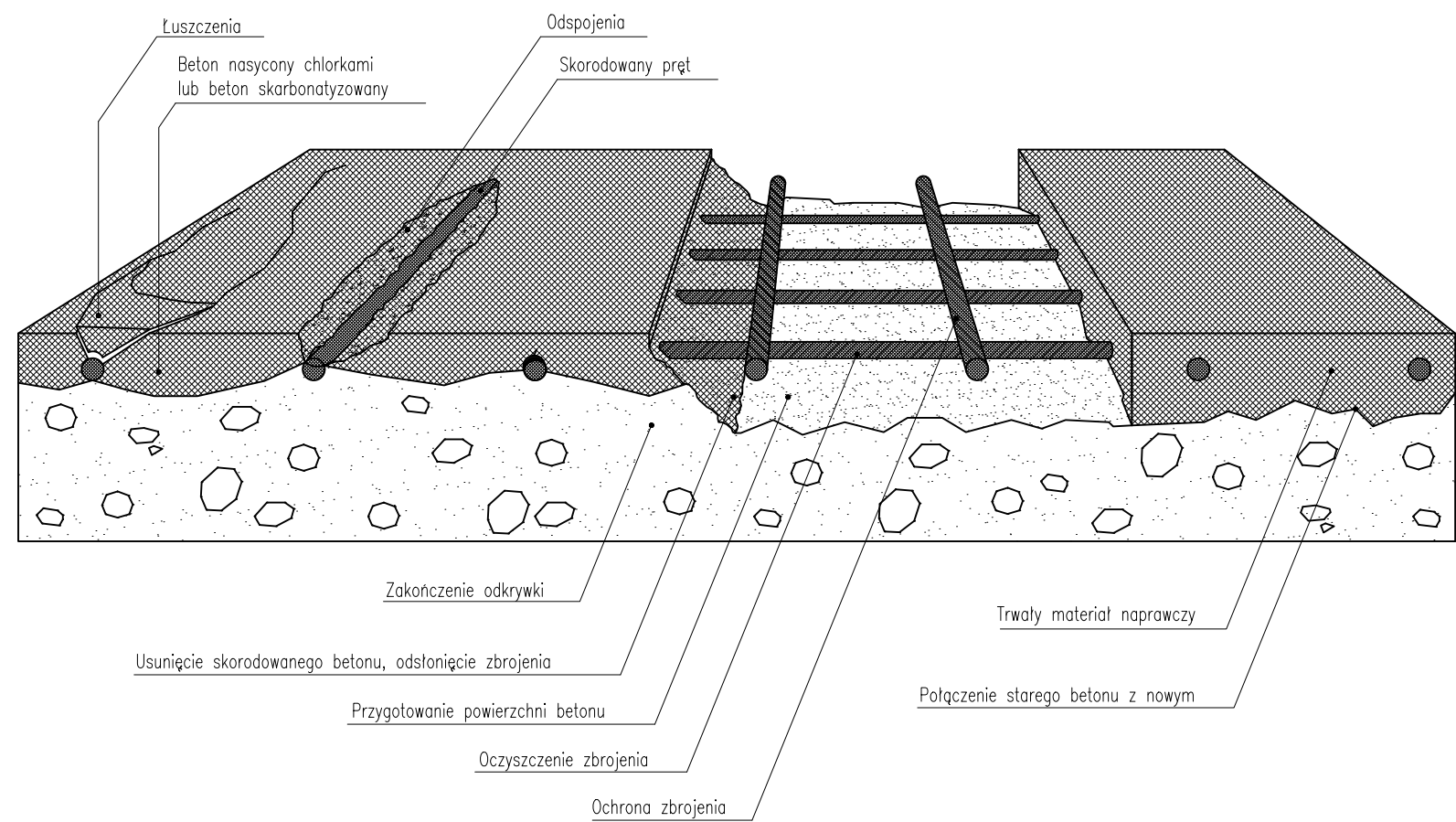
Przekrój pionowy przez płytę żelbetową
